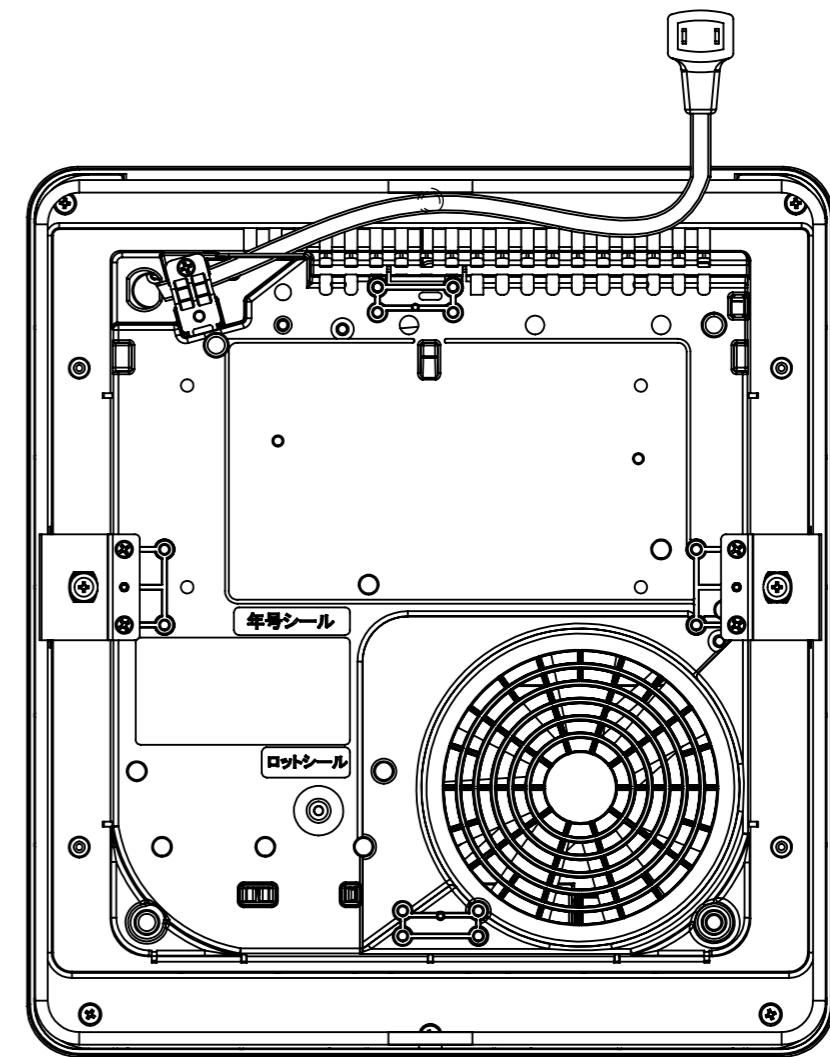
底面図
