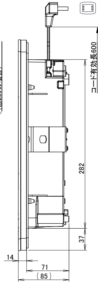
側面図
