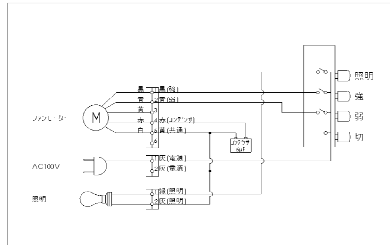
□ 結線図
