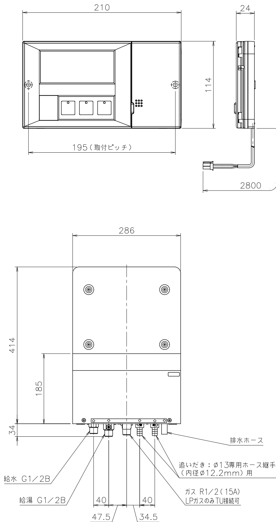
浴室リモコンRC-4026S (尺度1/3)
