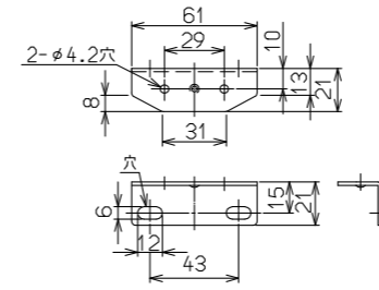
取付金具下(左右共通) 尺度: フリー
