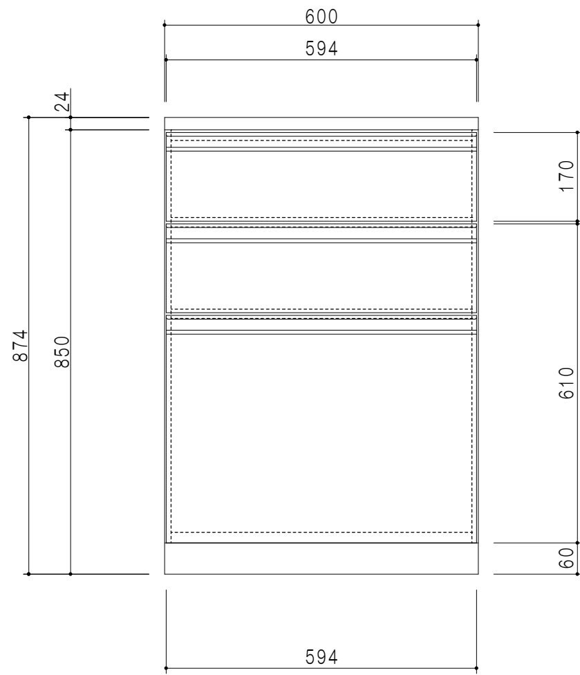
立面図
