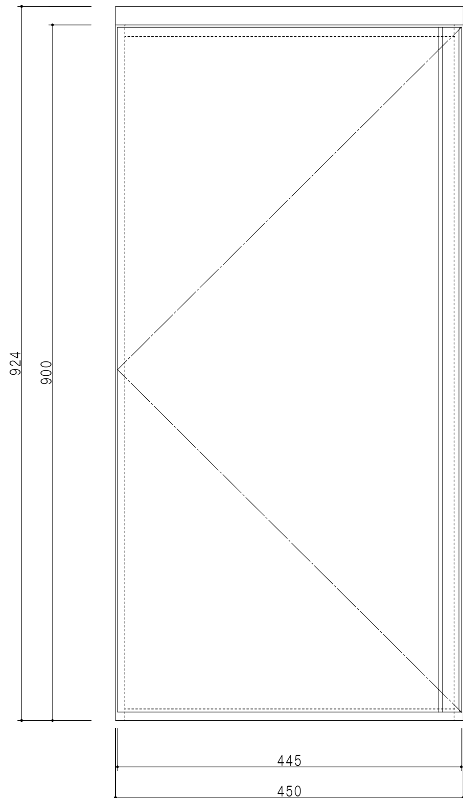
立面図
