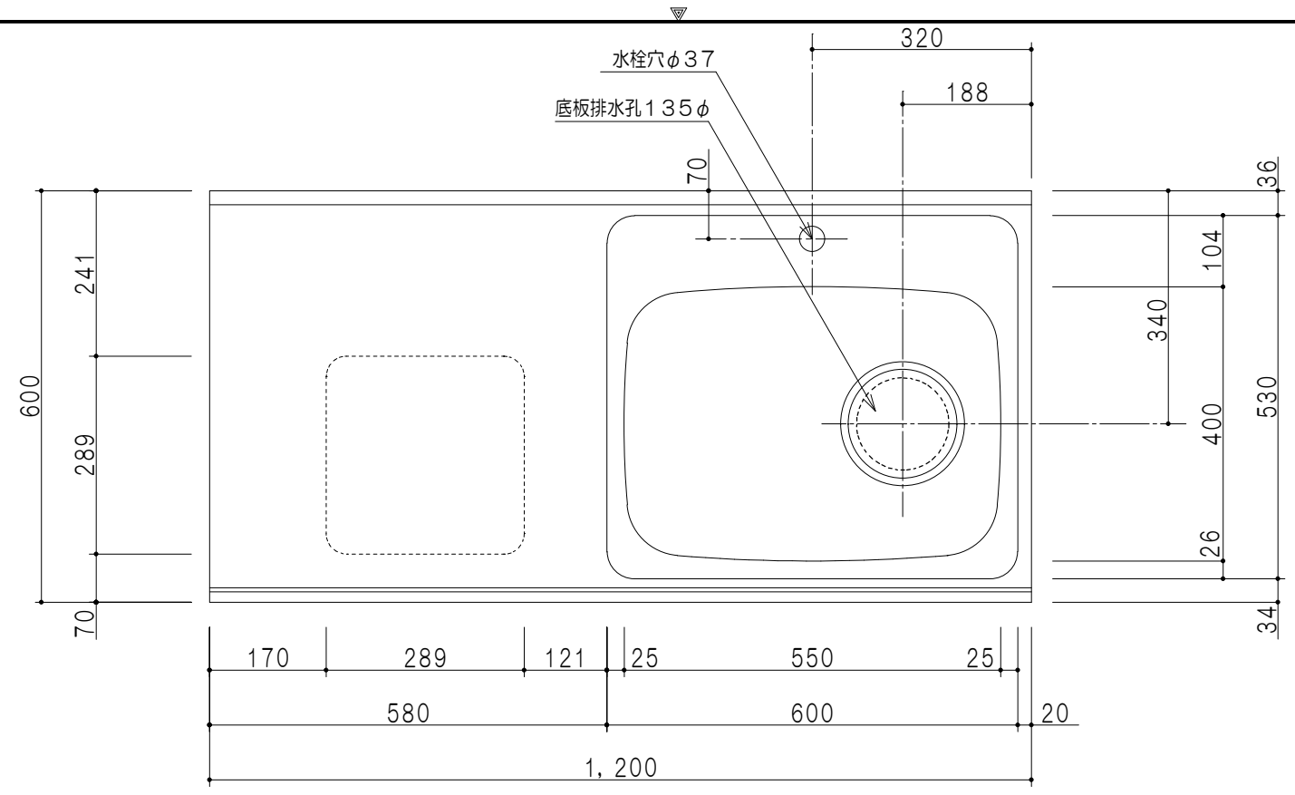
平面図
