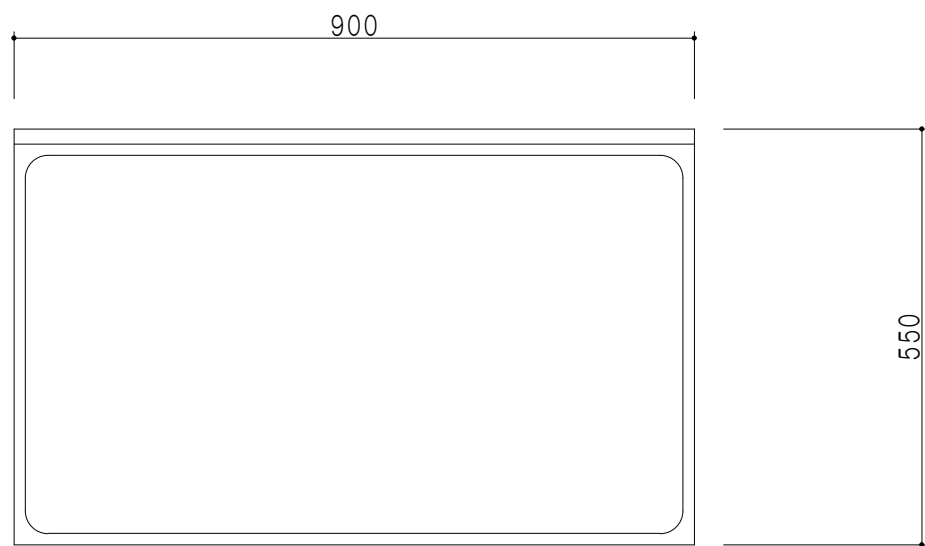
平面図
