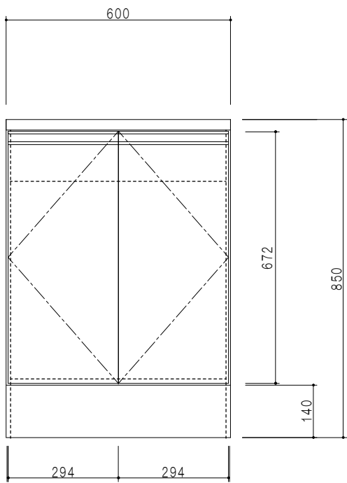
立面図
