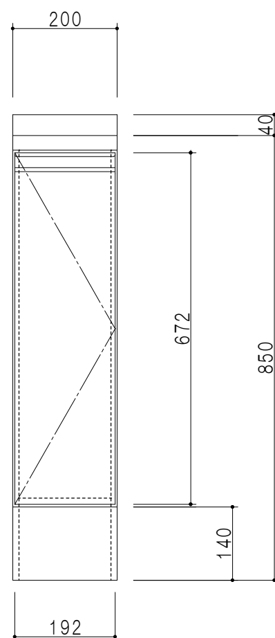
立面図
