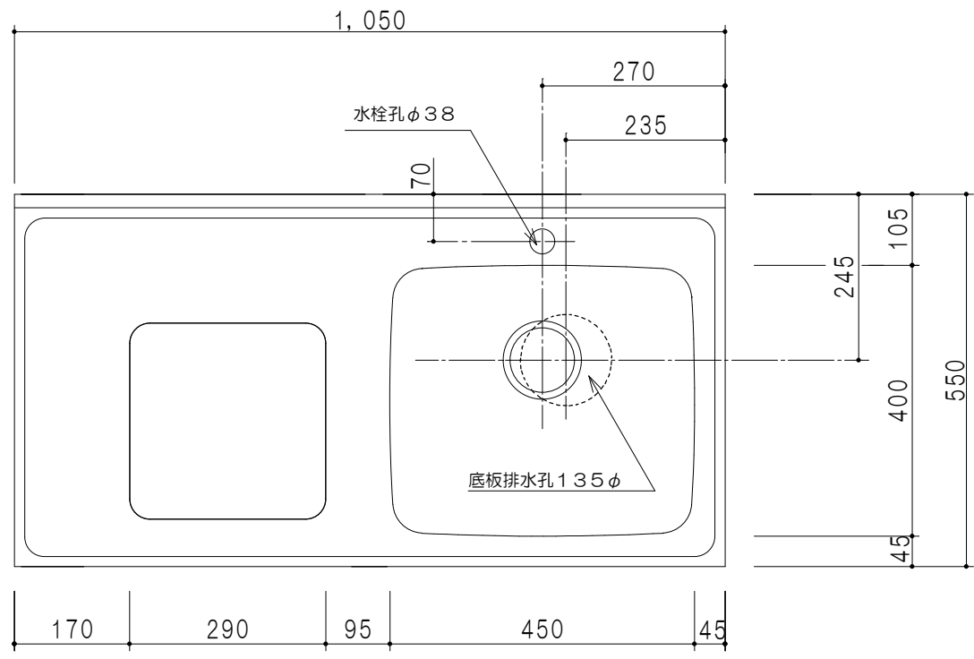
平面図
