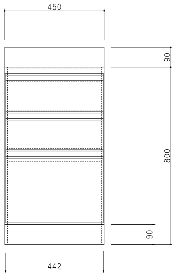
立面図
