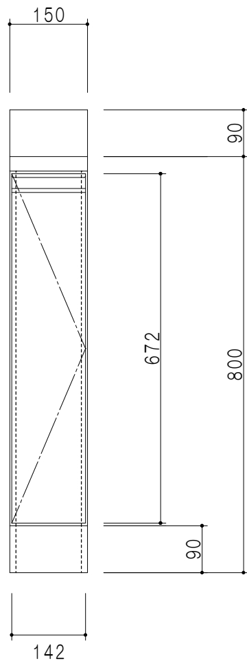
立面図
