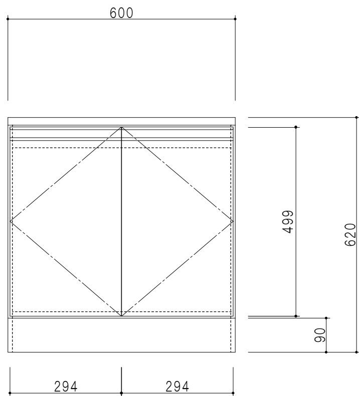
立面図
