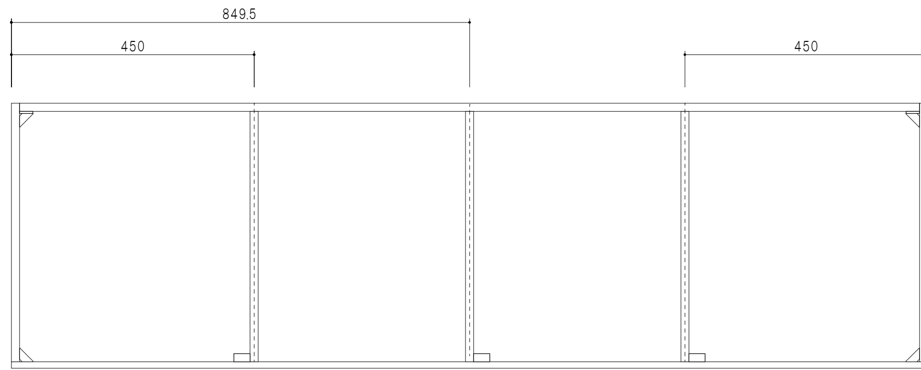
平面図
