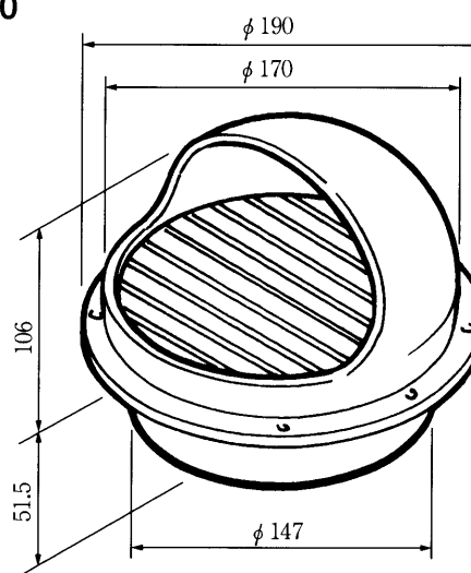
パイプフード150 (受注生産品) DFO-150
