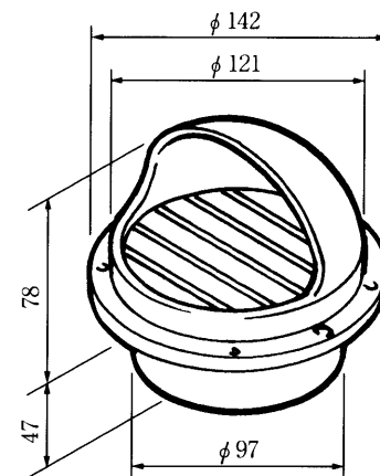
パイプフード125 DFO-125
