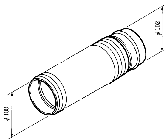
切替ダンパー接続フレキ管セット DFS-K100 (RDO-40BH)
