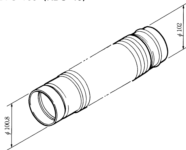
フレキ管セット DFS-100 (RDO-40)
