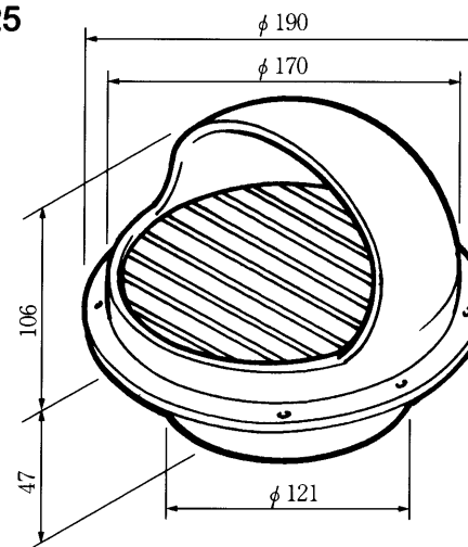
パイプフード150 (受注生産品) DFO-150
