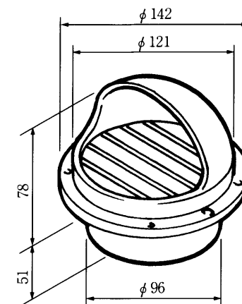
パイプフードF125 DFO-125F
