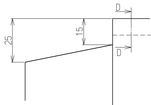
詳細図 A
