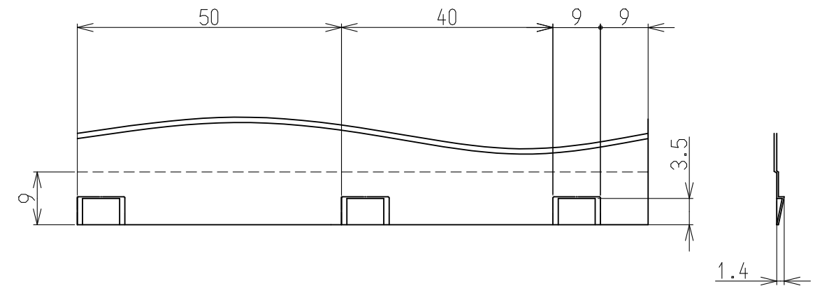
詳細図 C
