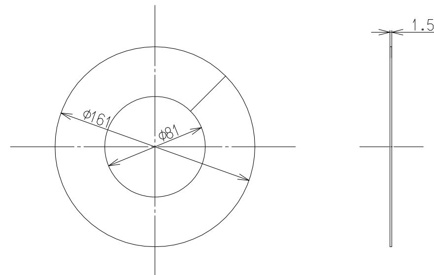
排湿管メガネリング(φ80)
