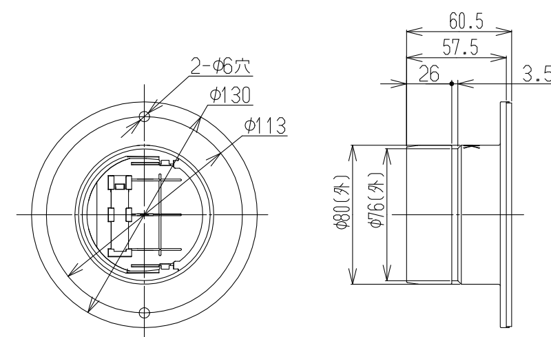
ダンパー付排湿口ガイド(φ80)
