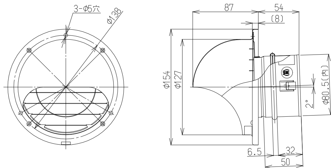
パイプフード(φ80)
