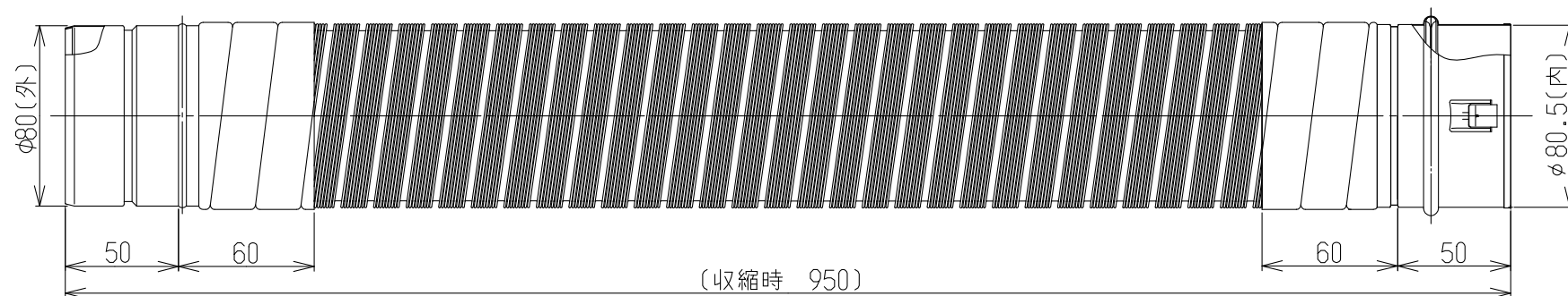
簡易排湿管(φ80)
