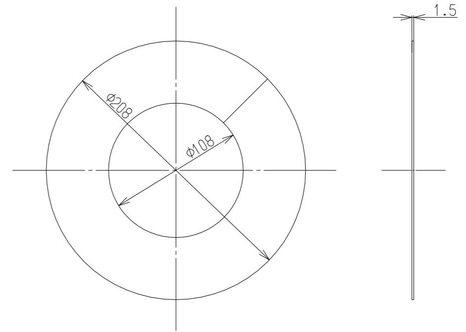
排湿管メガネリング(φ100)
