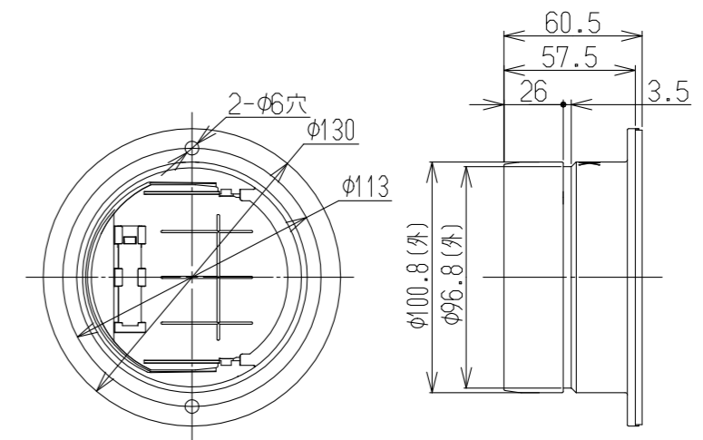
ダンパー付排湿ロガイド(φ100)
