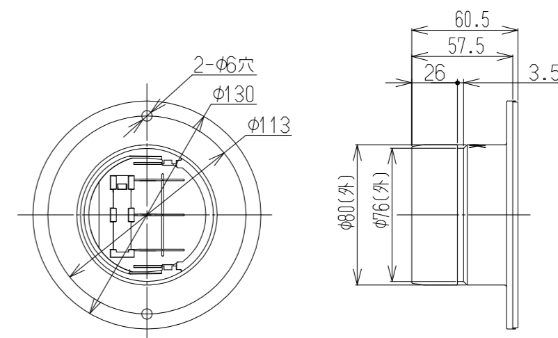
ダンパー付排湿ロガイド(φ80)
