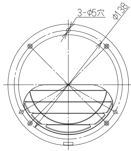
パイプフード(φ100)
