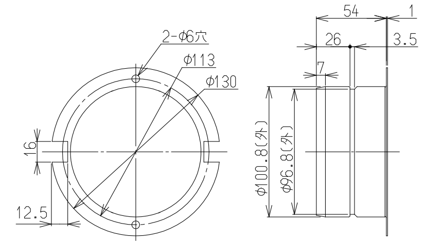
排湿口ガイド(φ100)
