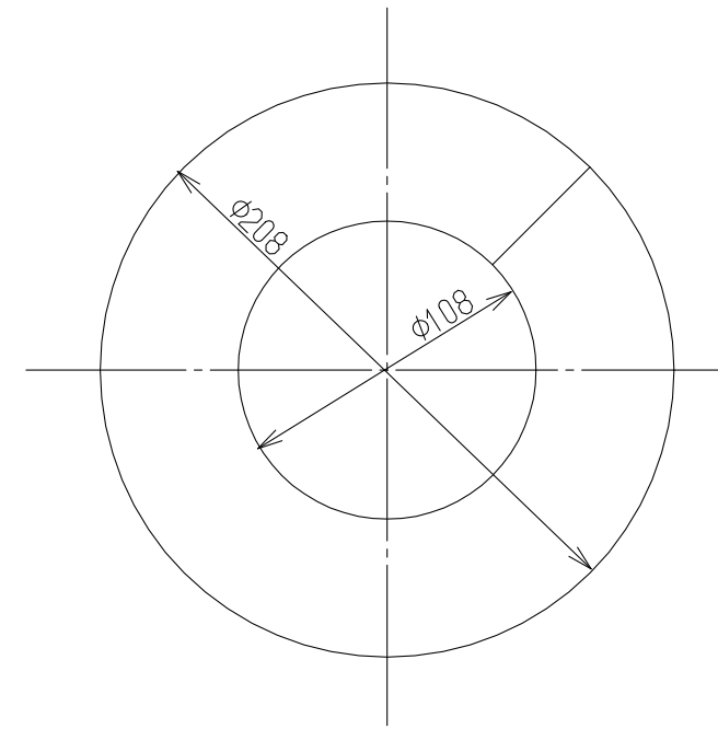
排湿管メガネリング(φ100)
