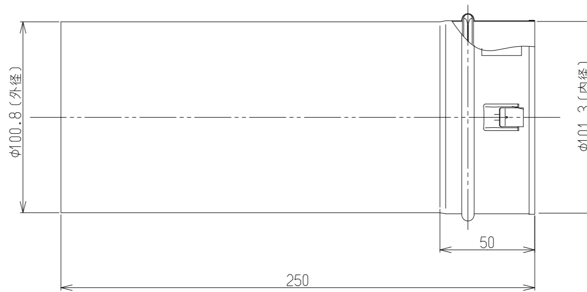
φ100アダプター
