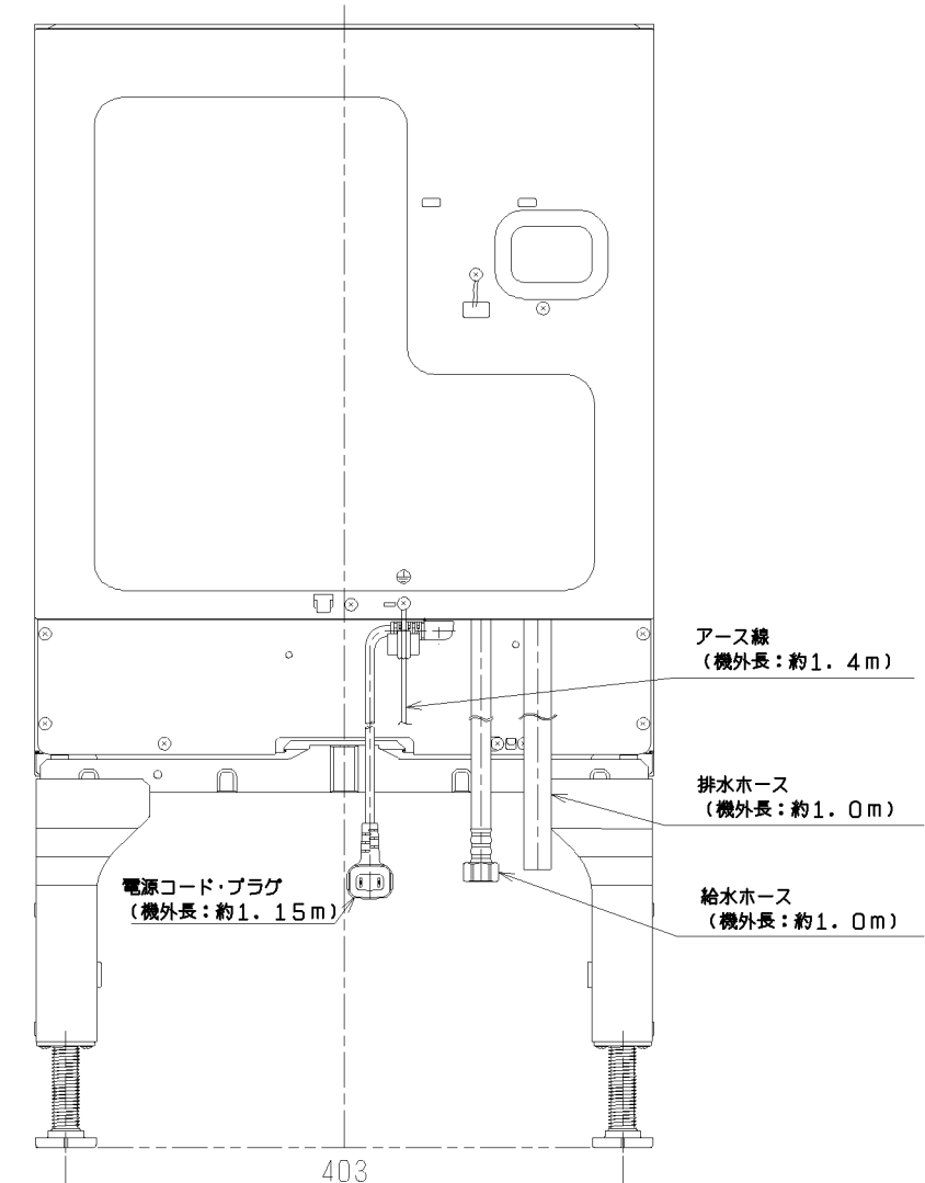
【背面図】
