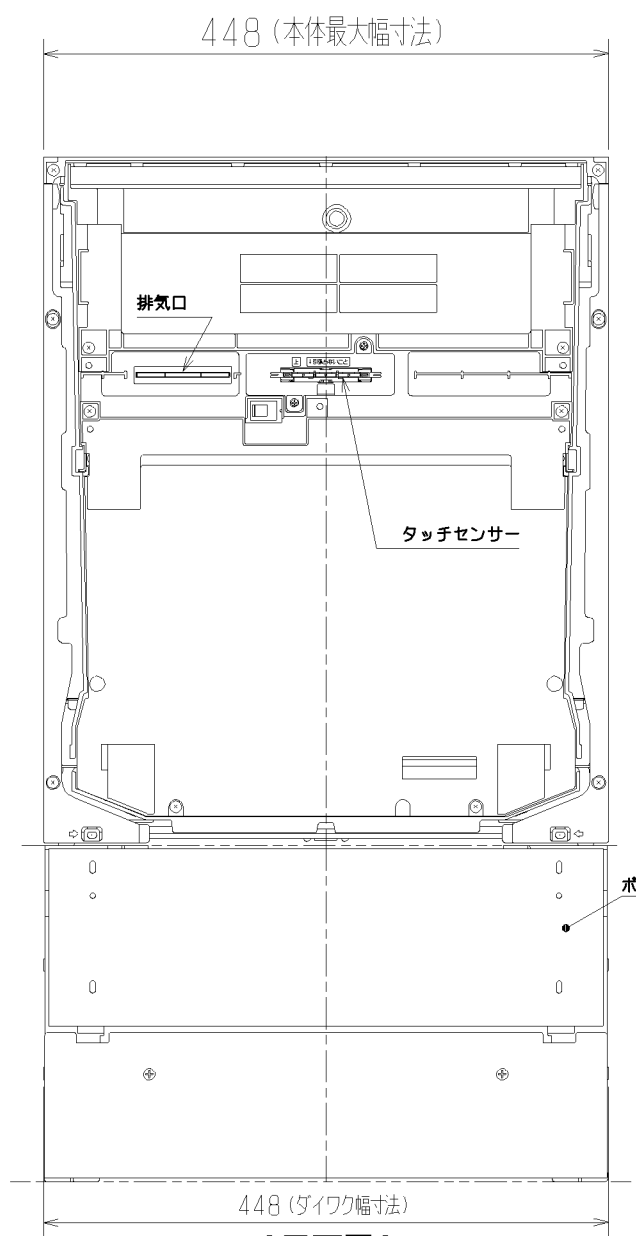
【正面図】
