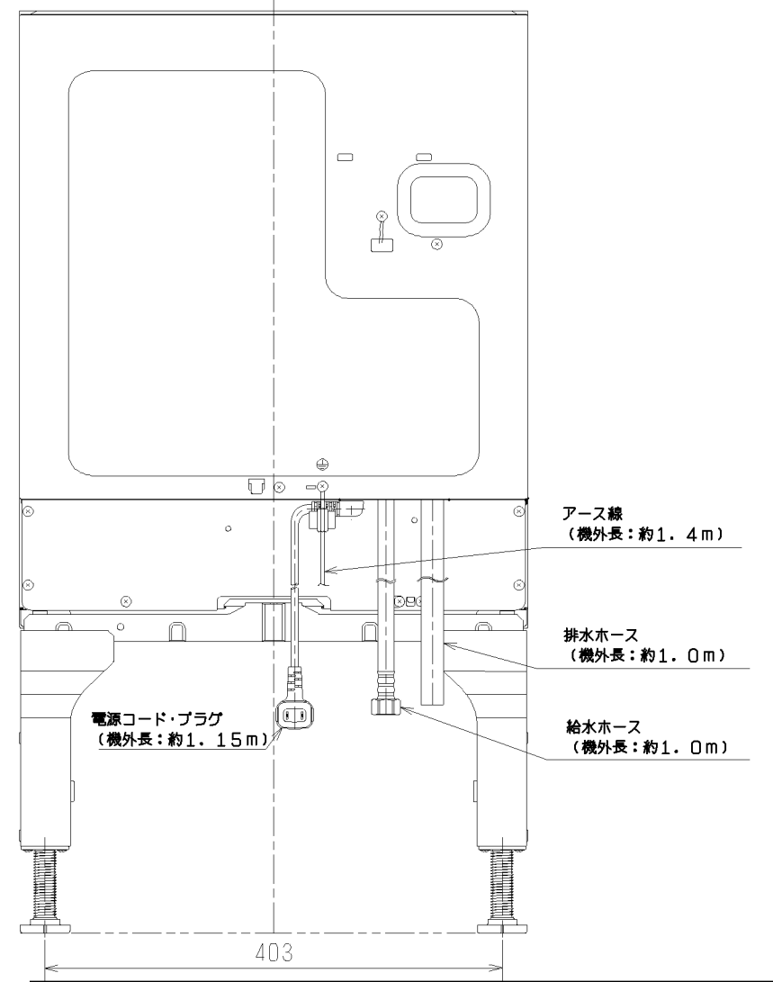
【背面図】
