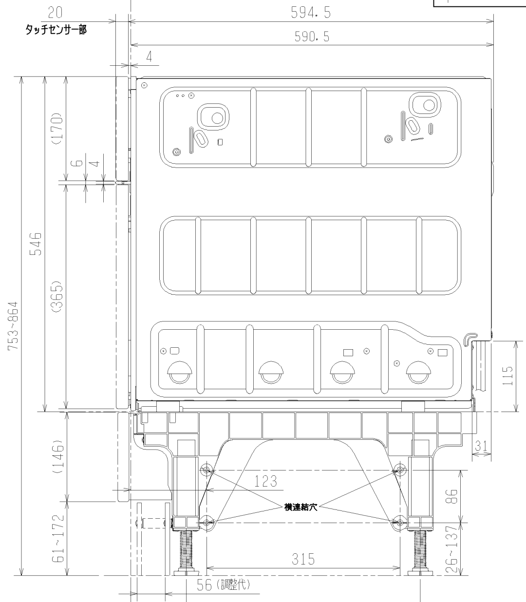
【側面図】
