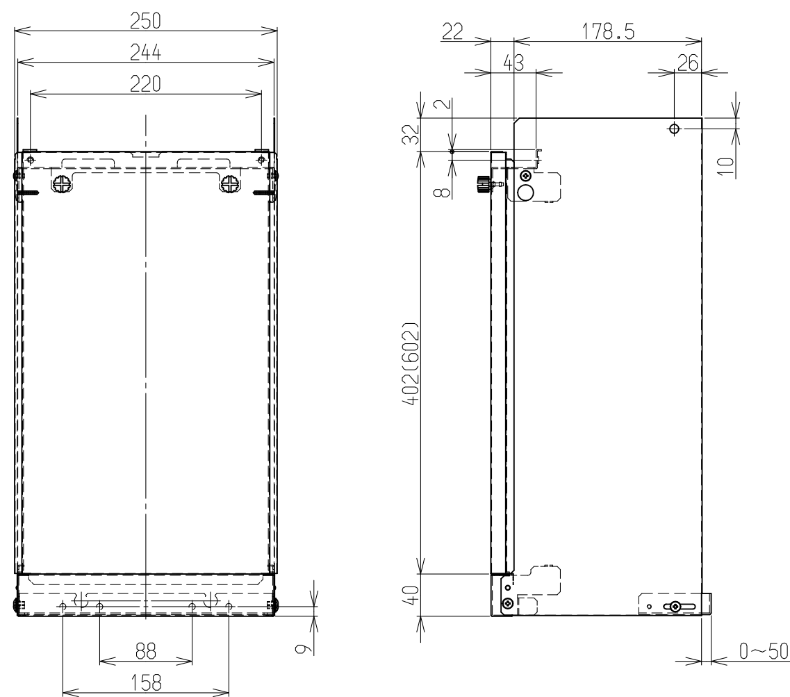
配管カバー寸法図
