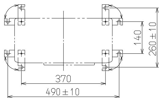
アンカーボルト位置図 [据置台固定金具(別売)を使用の場合]
