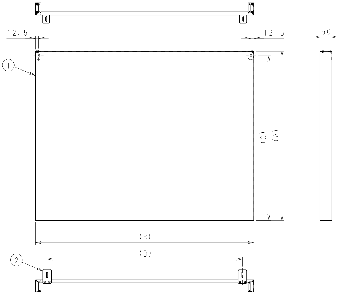
■寸法表
