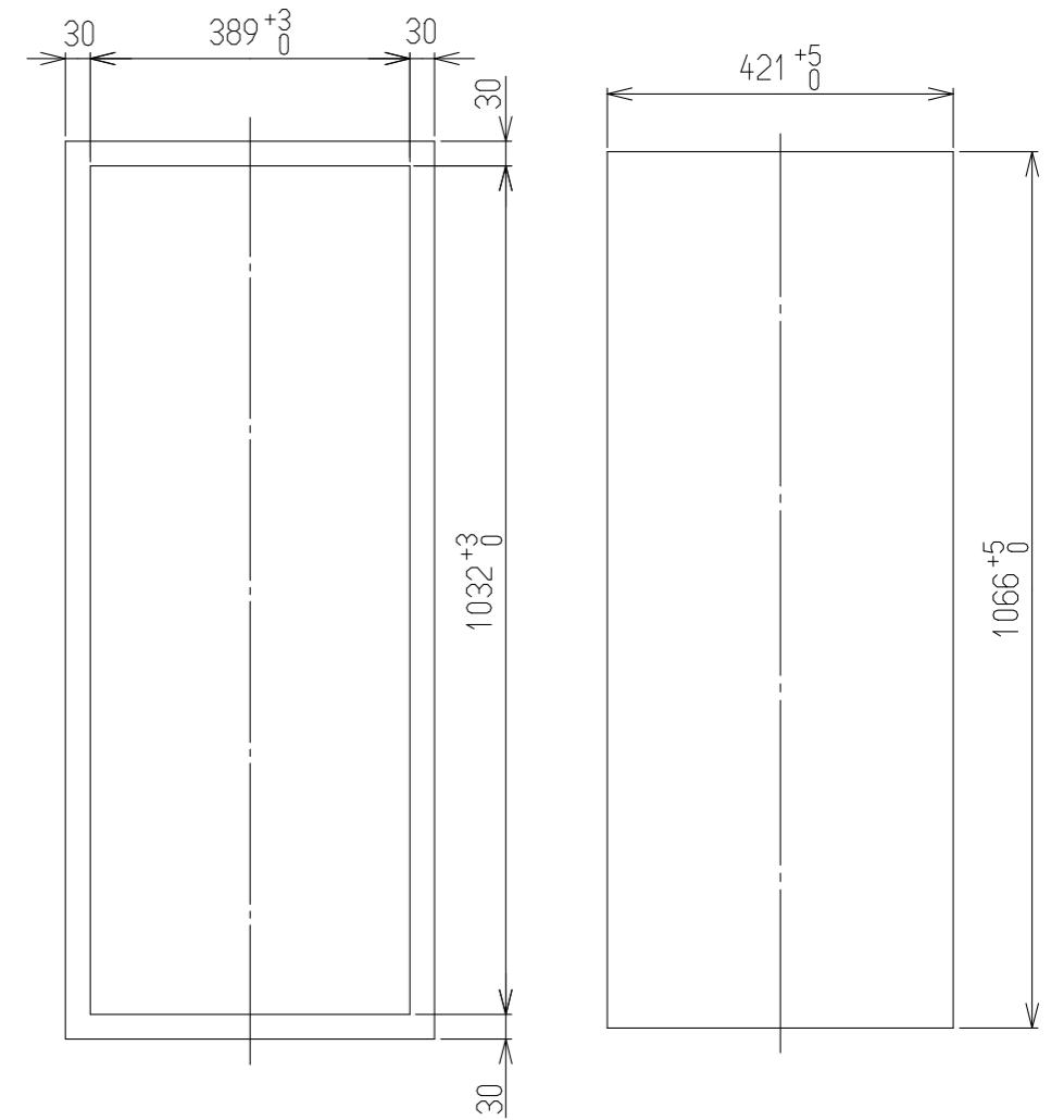
取付木枠寸法 (建築側準備)
