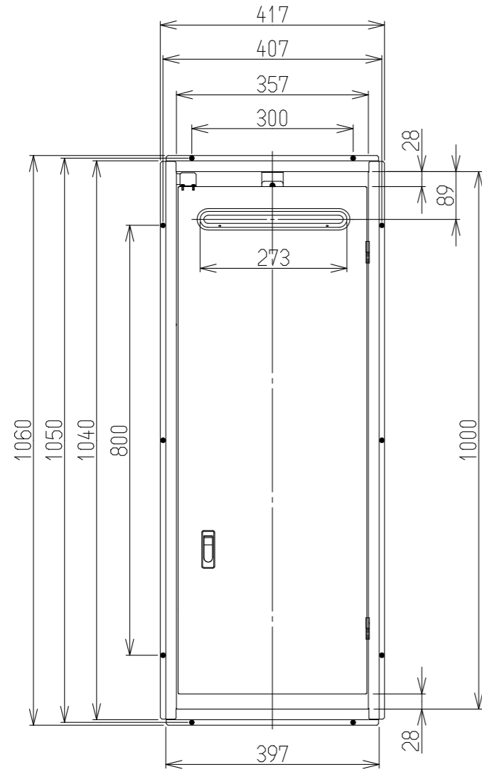
設置納まり図
