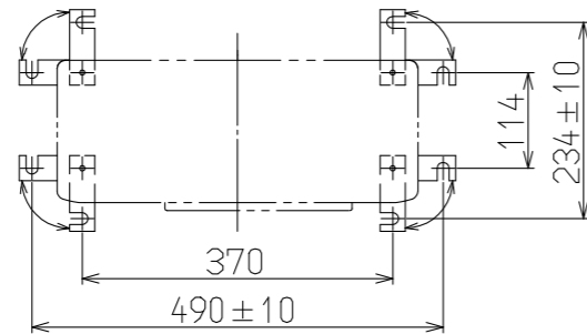
アンカーボルト位置図 (本体固定板使用の場合)
