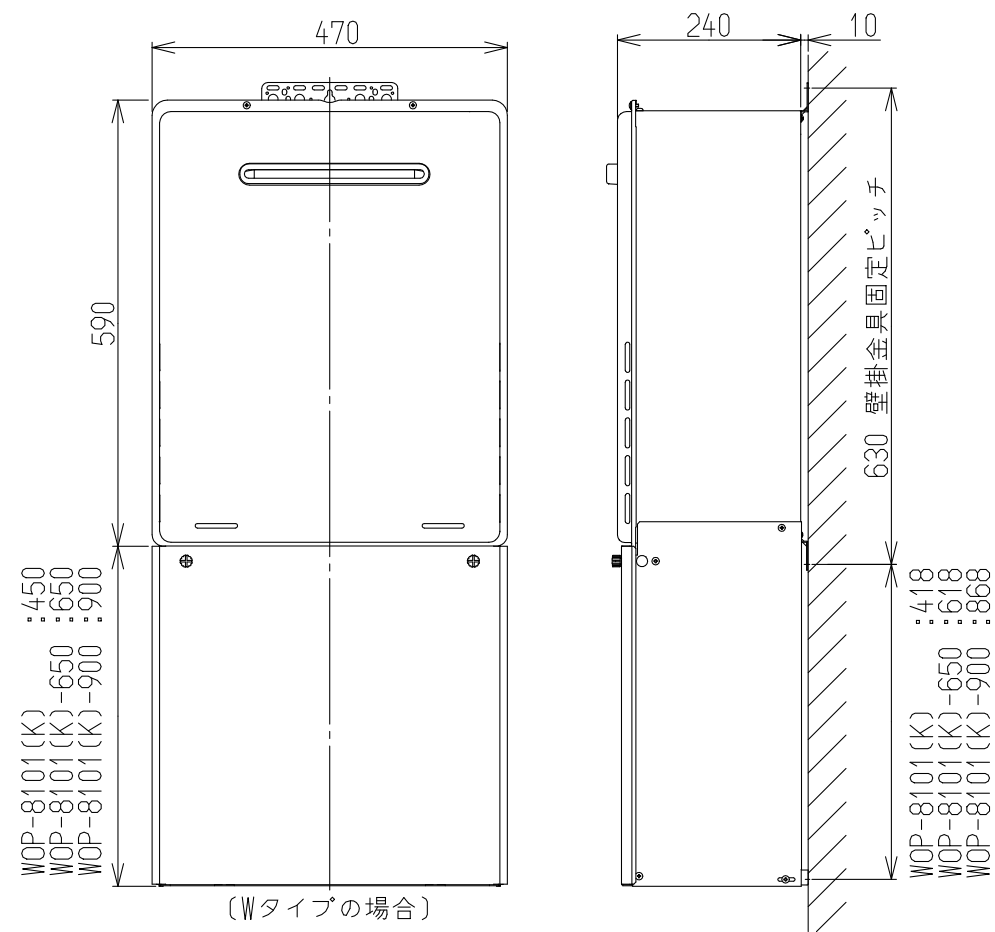
設置図 (S=1:10)
