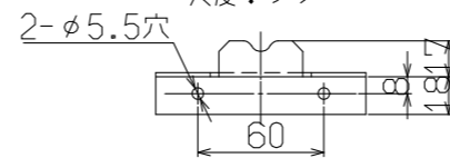
取付金具下(左右共通) 尺度:フリー
