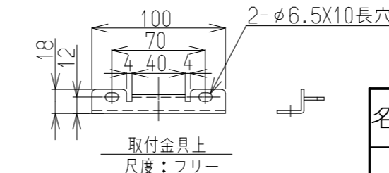
取付金具上 尺度:フリー
