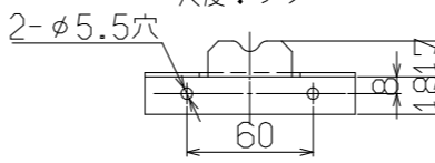
取付金具下(左右共通) 尺度:フリー
