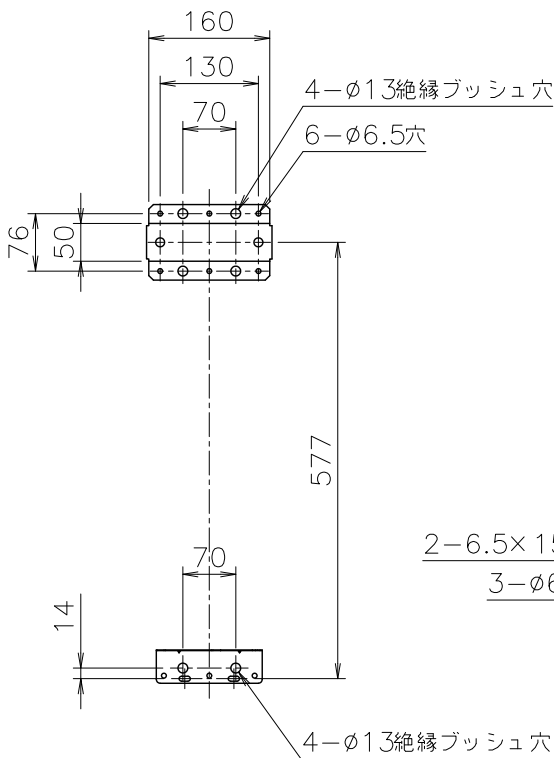
参 考 （壁掛金具 AGV使用時）
