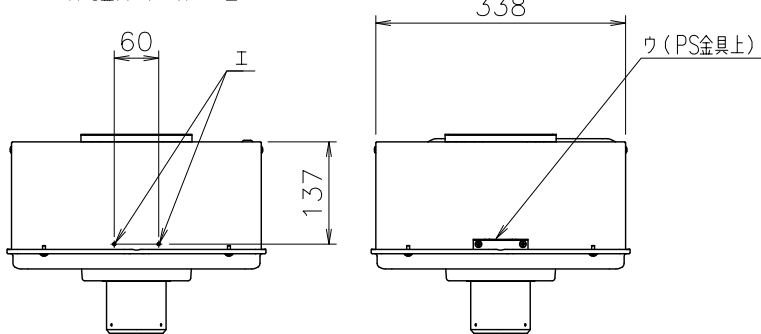
ウ（PS金具上）を外した図
