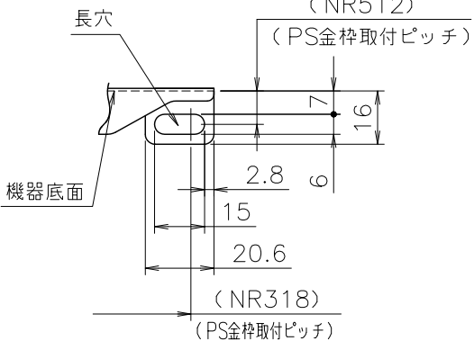
■イ部詳細（S=1/2）
