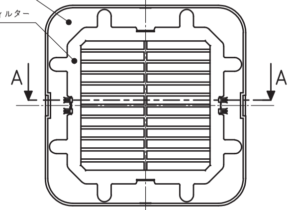
フィルター取付状態 (グリル裏面視)
