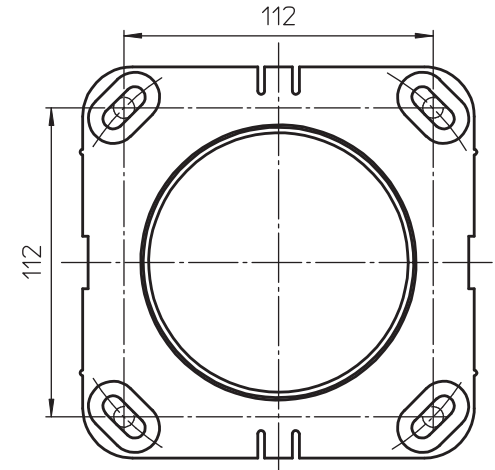
モリーアンカー取付寸法図 (裏面視)
