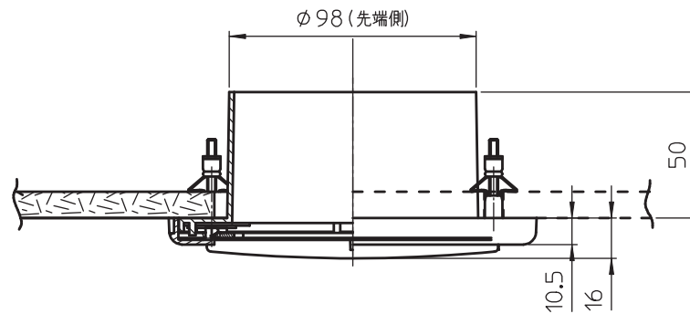
副吸込グリルフロント
